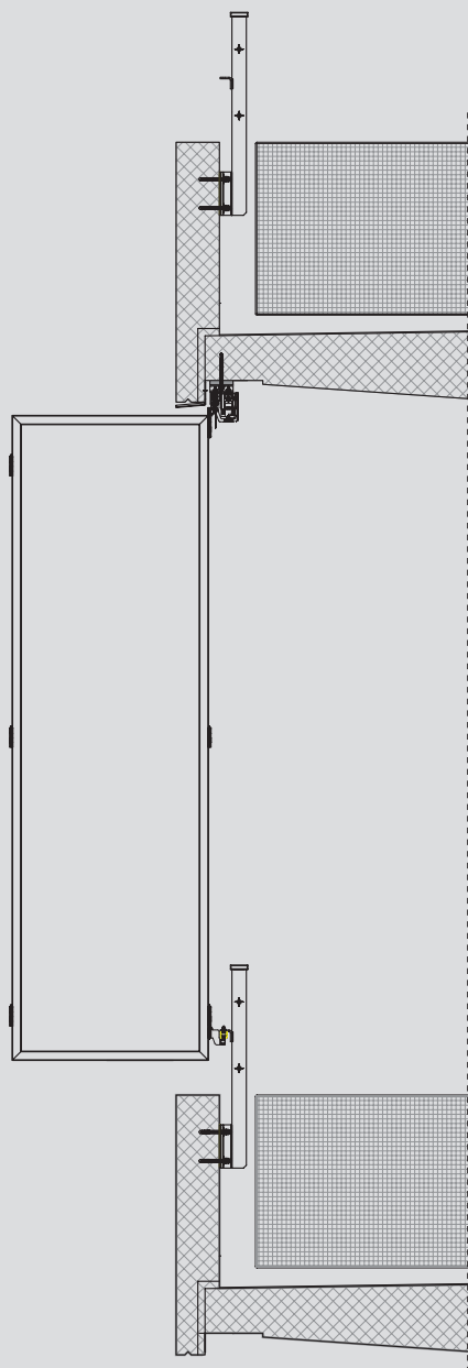
Vertikalschnittzeichnung
